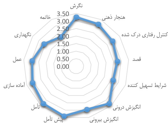
شکل ۲. میانگین‌های متغیرها
